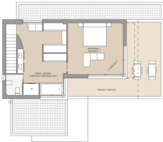
PLANTA PRIMERA | FIRST FLOOR
