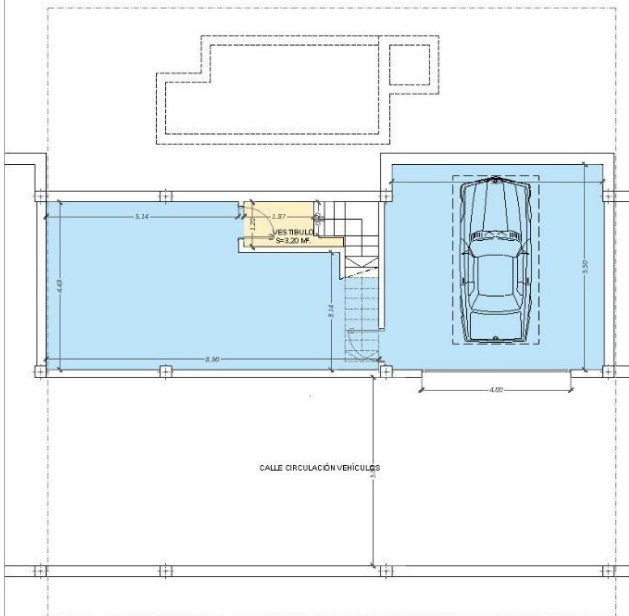
PLANTA SOTANO
