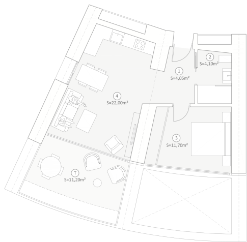
PLANTA 21
