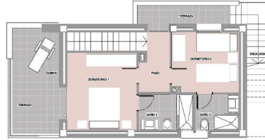
PLANTA PRIMERA
