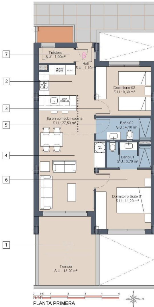
PLANTA PRIMERA
